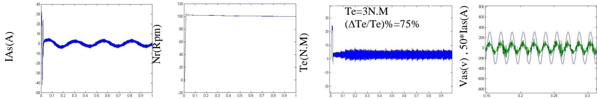
شکل(۶): نتایج کنترل سرعت 100 RPM به روش کنترل مستقیم گشتاور کلاسیک با مبدل ماتریسی 18 سوئیچ
