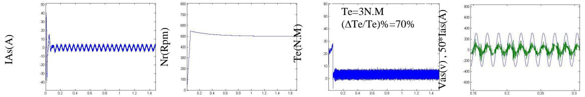
شکل(۷): نتایج کنترل سرعت 500 RPM به روش کنترل مستقیم گشتاور کلاسیک با مبدل ماتریسی 18 سوئیچ
