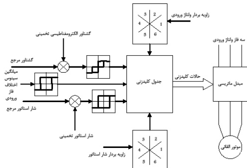
شکل (۲): کنترل مستقیم گشتاور با مبدل ماتریسی
