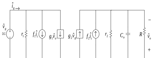
شکل (۷): مدار معادل مدل سیگنال کوچک اصلاح کننده ضریب توان بر پایه مبدل شپارد-تیلور
