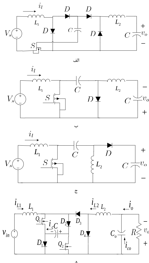
شکل (۱): توپولوژی های تک مرحله مبدل های باک بوست (الف) مبدل باک بوست آبشاری (ب) مبدل چوک (ج) مبدل سپیک (د) مبدل شپارد-تیلور [۸]
