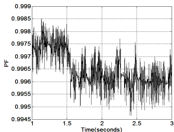
شکل (۱۷): ضریب توان جریان ورودی در حین تغییر پله ای بار کامل به نصف بار کامل
