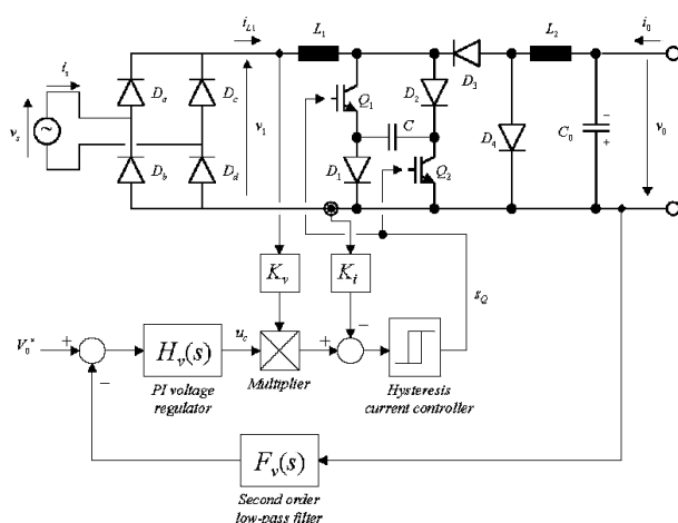
شکل (۱۹): سیستم کنترلی هیستریزیس [۸]
