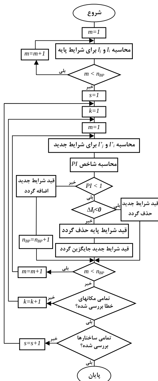
شکل (۱): الگوریتم پیشنهادی به منظور اعمال شاخص پیشنهادی به مساله هماهنگی رله های اضافه جریان با در نظر گرفتن عدم قطعيتها
