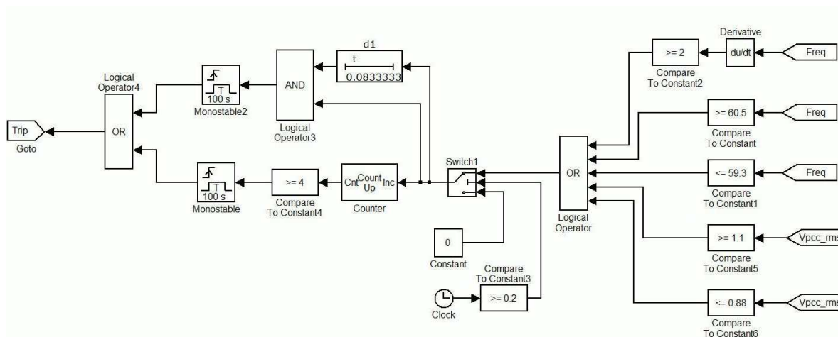
شکل (۳): سیستم حفاظتی و تشخیص حالت جزیره‌ای با استفاده از روش ترکیبی رله های OVP / UVP ، OFP / UFP و ROCOF.
