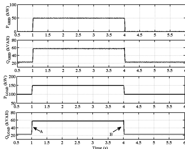
شکل (۶): شرایط شبکه و بار در زمان بهره برداری نرمال شبکه
