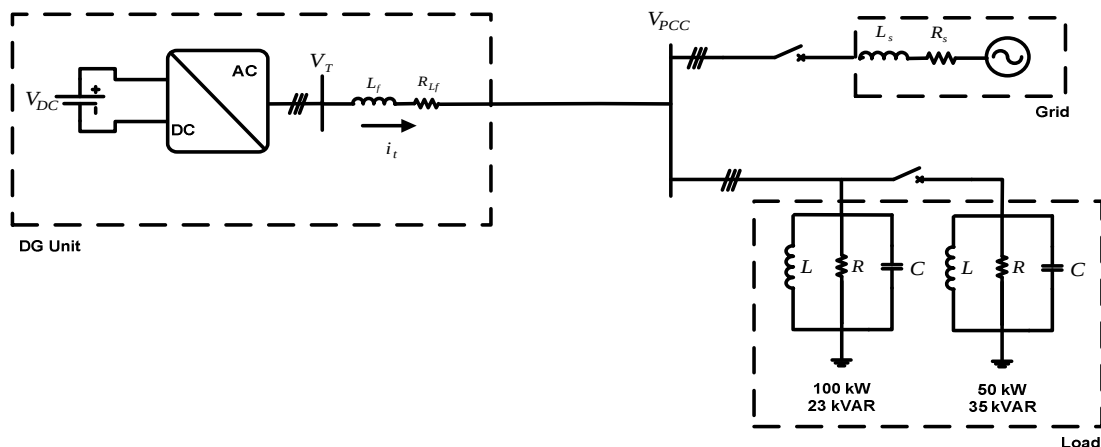
شکل (۴): سیستم مورد مطالعه
