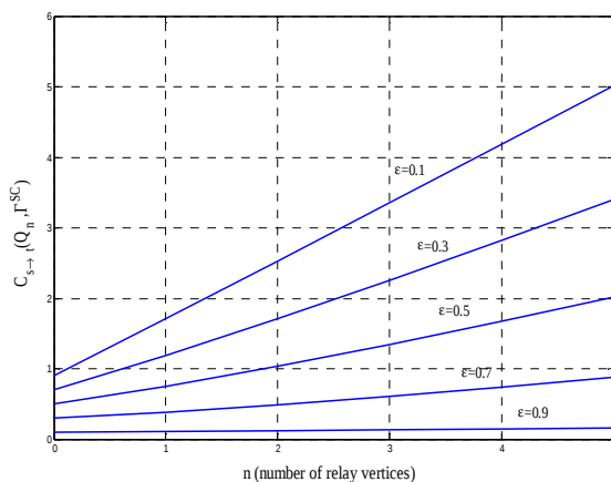
شکل (۱۱): ظرفیت تحت کدینگ فضایی شبکه برای \varepsilon های مختلف
