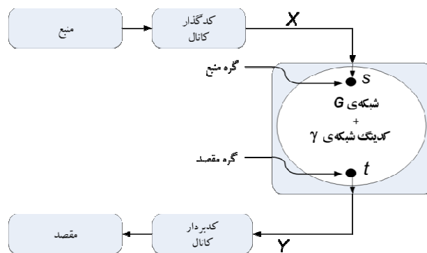
شکل (۲): دیگرام بلوکی یک سیستم مخابراتی که در آن شبکه‌ی G به عنوان کانال مخابراتی بین گره‌ی منبع S و گره‌ی مقصد t عمل می‌کند.
