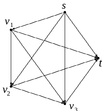
شکل (۹): گراف G_3^*
