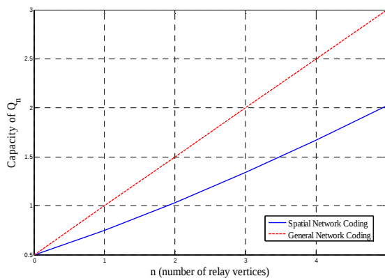
شکل (۱۰): مقایسه بین ظرفیت تحت کدینگ فضایی شبکه و کدینگ عام شبکه برای \varepsilon = 0.5
