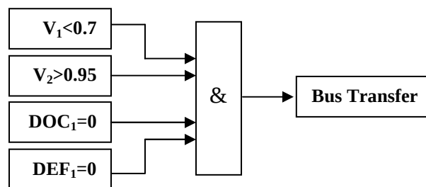
شکل (۸): منطق کنترلی پیشنهادی برای انجام انتقال سریع باس بجای روش متداول استفاده از کنتاکتهای کمکی کلید
