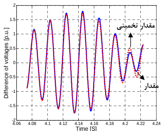
شکل (۱۵): ولتاژهای واقعی و تخمینی دو سر کلید CB2
