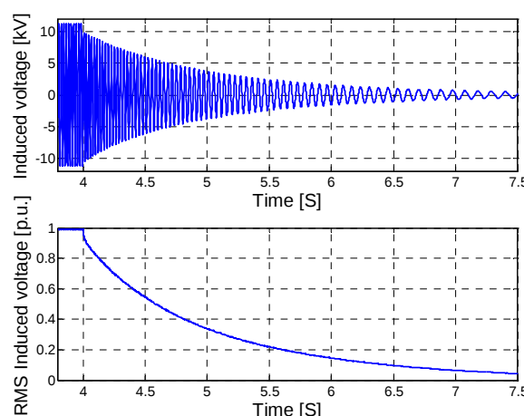
شکل (۳): شکل موج و مقدار موثر ولتاژ القایی در ترمینال موتور مورد مطالعه پس از قطع ولتاژ تحریک
