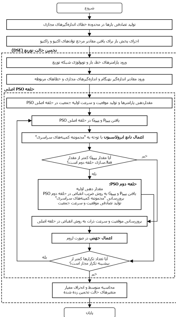
شکل (۴): فلوچارت DSE بر مبنای الگوریتم پیشنهادی DLM-PSO
