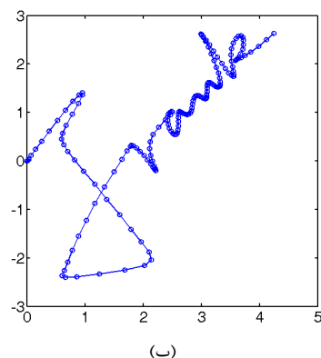
شکل (۳): برازش خطی و اصلاح خط مبنا. (الف) - الگوی اولیه. (ب) - پس از اصلاح زاویه ترسیم.
