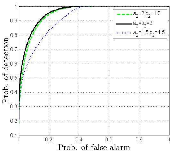
شکل (۱): نمودار احتمال آشکارسازی در برابر احتمال هشدار غلط برای آشکارساز UMPI به ازای سه مقدار a_2 = b_2 = 2 و a_2 = 2, b_2 = 1.5 و a_2 = 1.5, b_2 = 1.5 برای فرضیه H_1 در برابر H_0 به ازای فرضیه H_0
