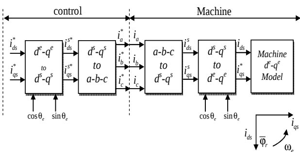
شکل (۱): بلوک دیاگرام کنترل برداری مدل d-q موتور القایی [1].
