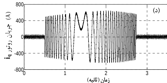
شکل (۶): نتایج شبیه سازی برای سرعت 1000 \text{ rpm} \pm بدون جبران شار روتور، الف: پروفایل سرعت روتور، ب: پروفایل گشتاور تولیدی، ج: جریان روتور بر روی محور d و د: جریان روتور بر روی محور q
