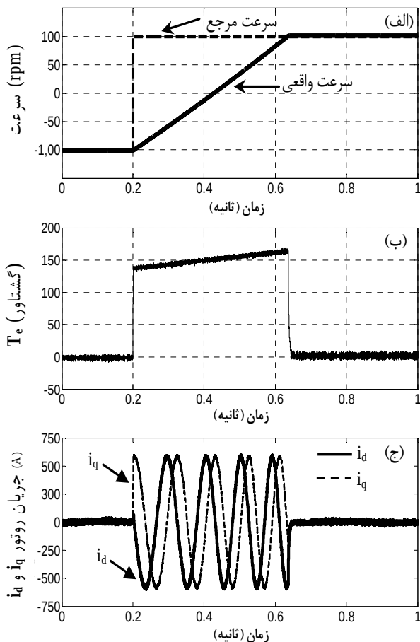
شکل (۸): نتایج شبیه‌سازی برای سرعت 100 \text{ rpm} \pm با جبران‌ساز شار روتور، الف: پروفایل سرعت روتور، ب: پروفایل گشتاور تولیدی، ج: مؤلفه‌های جریان روتور در قاب dq .
