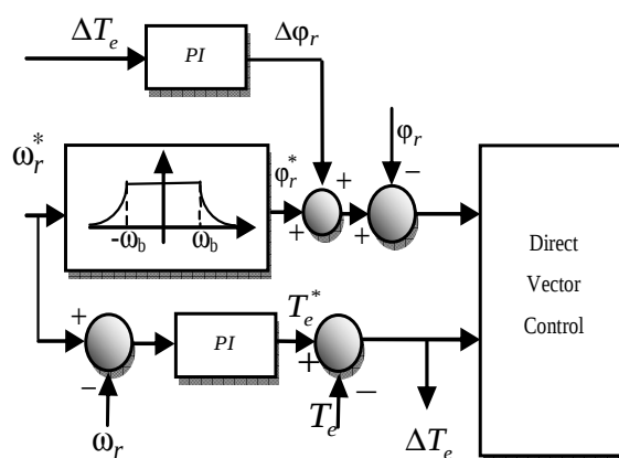
شکل (۵): بلوک دیاگرام مربوط به جبران شار روتور.
