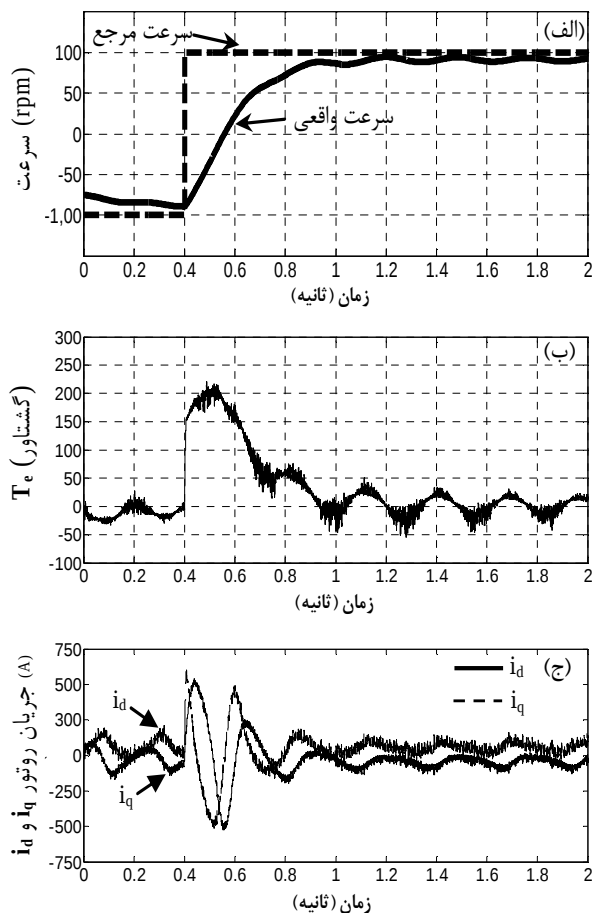
شکل (۷): نتایج شبیه‌سازی برای سرعت 100 \text{ rpm} \pm بدون جبران شار روتور، الف: پروفایل سرعت روتور، ب: پروفایل گشتاور تولیدی و ج: مؤلفه‌های جریان روتور در قاب dq .
