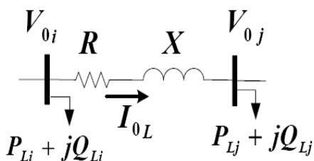
شکل (۲): دیاگرام تک خطی یک سیستم توزیع ۲ باسه
