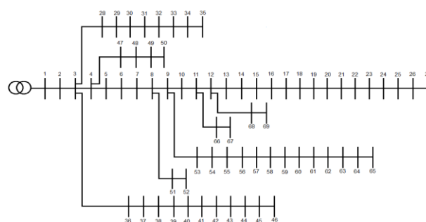
شکل (۹): دیاگرام تک خطی شبکه توزیع ۶۹ باسه IEEE
