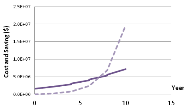
شکل (۱۱): منحنی بازگشت سرمایه شبکه ۶۹ باسه برای ۵ پله بار در طی ۱۰ سال (—Cost, ---Saving)
