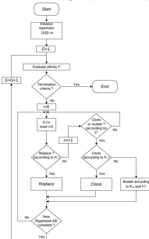
شکل (۶): فلوچارت الگوریتم ایمنی
