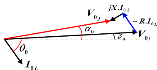
شکل (۳): دیاگرام فازوری ولتاژ و جریان سیستم توزیع شکل (۲)
