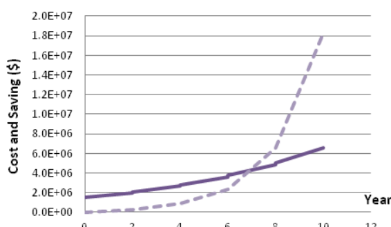
شکل (۱۰): منحنی بازگشت سرمایه شبکه ۳۳ باسه برای ۵ پله بار در طی ۱۰ سال (—Cost, ---Saving)
