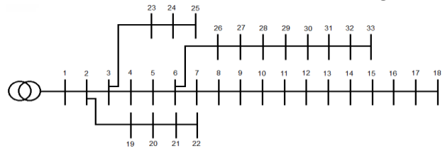
شکل (۸): دیاگرام تک خطی شبکه توزیع ۳۳ باسه IEEE
