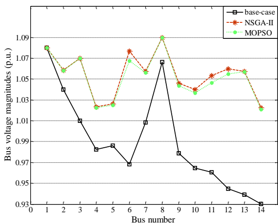
شکل (۱۰): دامنه ولتاژ باس‌ها به ازای حالت اولیه در مقایسه با نتایج
