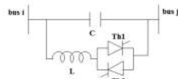
شکل (۱): ساختار TCSC
