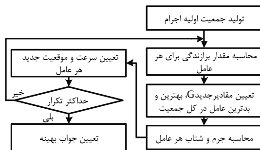
شکل (۱): فلوچارت الگوریتم جستجوی گرانشی
