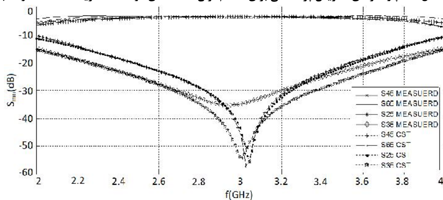
شکل (۱۲): پارامترهای ماتریس پراکندگی برای مقسم توان ۶ دهانه ای در حالت تحریک دهانه (۵) و نسبت توان 1:1:1
