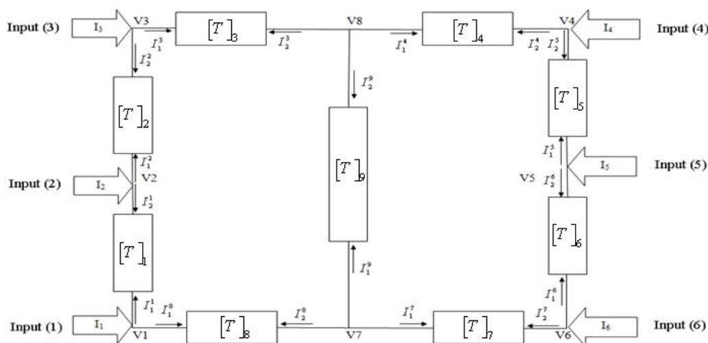
شکل (۴): ترکیب اجزای تفکیک شده مقسم توان ۶ دهانه ای
