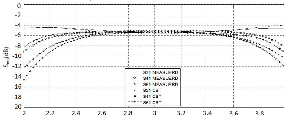
شکل (۷): پارامترهای ماتریس پراکندگی برای مقسم توان ۶ دهانه ای در حالت تحریک دهانه (۱) و نسبت توان 1:1:1
