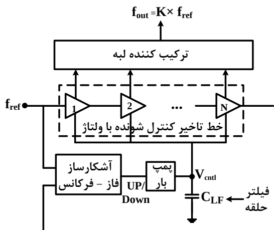
شکل (۱): ساختار یک ضرب کننده فرکانسی متداول براساس حلقه قفل شده تاخیر
