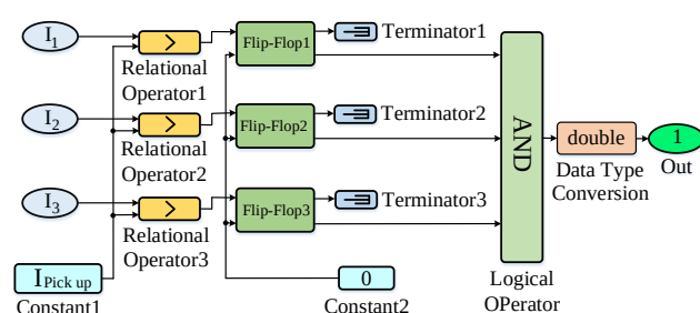
شکل (۵): منطق پیشنهادی برای پیاده‌سازی طرح ارائه شده
