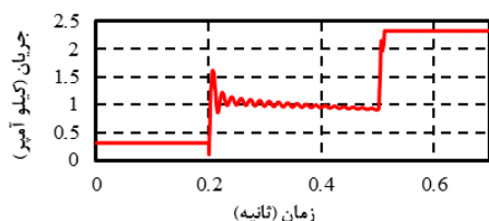
شکل (۳): جریان اتصال کوتاه دوسطی عبوری از رله R_{pr}
