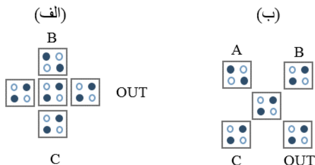
شکل (۶): ساختارهای موجود برای گیت اکثریت
