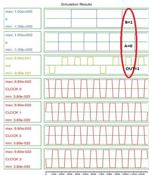
شکل (۱۲): نتیجه شبیه سازی گیت OR پیشنهادی
