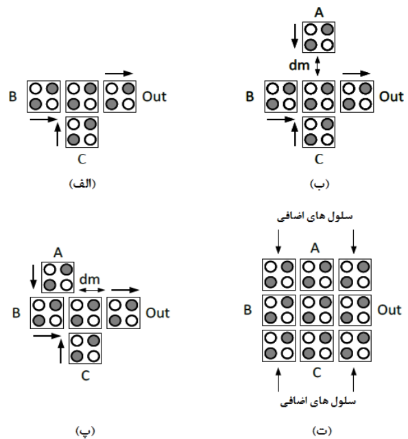
شکل (۷): انواع خطاهای احتمالی در QCA: (الف) خطای حذف سلول (ب) خطای جابجایی سلول (پ) خطای ناهمترایی سلول (ت) خطای رسوب سلول اضافی
