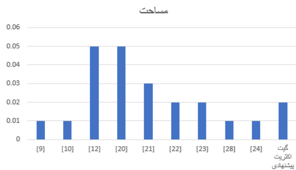
شکل (۱۴): نمودار مقایسه مساحت گیت اکثریت پیشنهادی (بر حسب \mu m^2 ) با بقیه کارها
