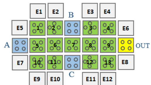
شکل (۱۳): سلول‌های اضافی اطراف گیت اکثریت سه ورودی پیشنهادی
