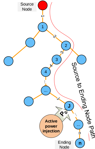
شکل (۱): شبکه‌ی توزیع شعاعی با تزریق توان اکتیو به گره j
