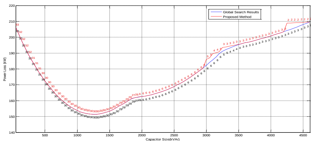
شکل (۴): تلفات توان محاسبه شده از روش پیشنهادی و روش جستجوی سراسری به ازای تزریق توان راکتیو به شبکه از ۱۰۰ کیلووار تا ۴۶۰۰ کیلووار
