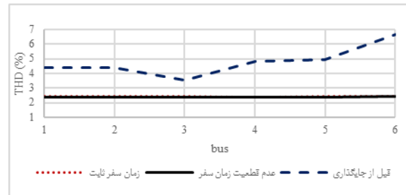
شکل (۴): THD باس‌ها در پیک تقاضای شبکه توزیع قبل و بعد از جایگذاری ایستگاه‌های شارژ سریع
