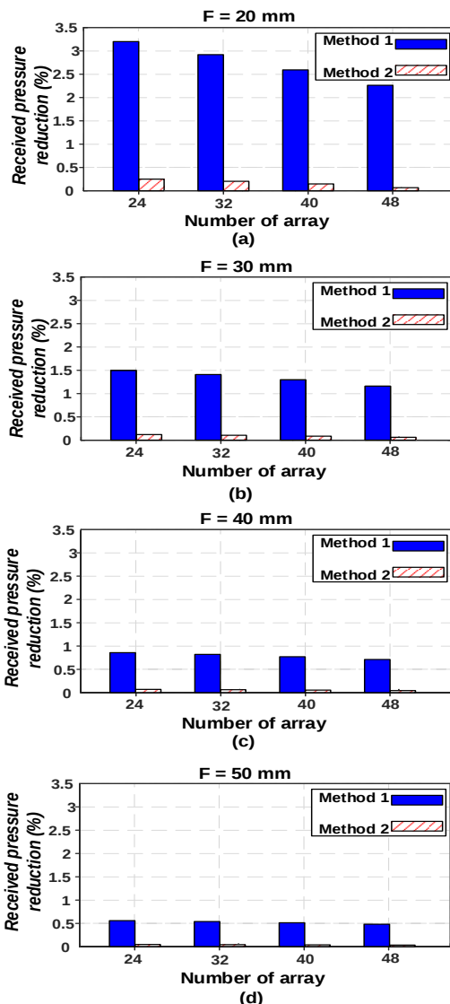
شکل (۵): کاهش فشار صوتی دریافتی برای روش پیشنهادی ۱ و ۲ و تعداد متفاوت عناصر آرایه برای (a) F=20\text{mm} (b) F=30\text{mm} (c) F=40\text{mm} (d) F=50\text{mm}
