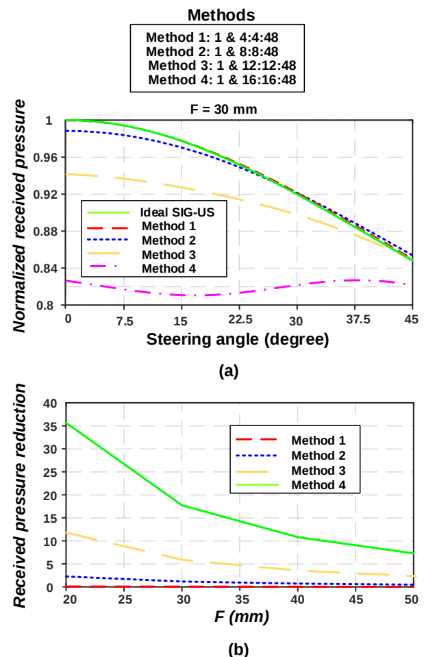
شکل (۶): (a) فشار نرمالیزه شده دریافتی برای N=48 و فاصله کانونی 30 \text{ mm} در برابر زاویه هدایت و چهار روش تخمین خطی، (b) کاهش فشار دریافتی در برابر فاصله کانونی ( F ) برای چهار روش پیشنهادی
