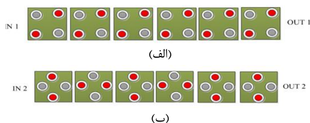
شکل (۲): نحوه اجرای متداول سیمها در تکنولوژی QCA
