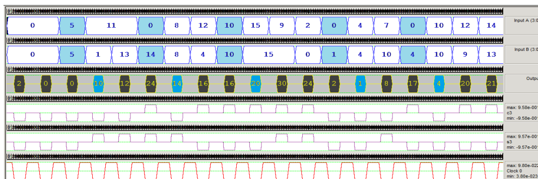
شکل (۹): نتایج شبیه‌سازی RCA ۴-بیتی پیشنهادی
