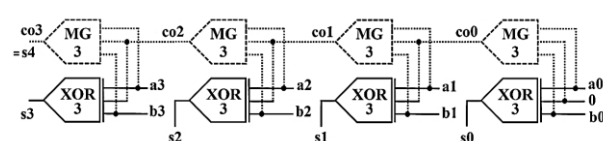
شکل (۶): بلوک دیاگرام جمع کننده RCA ۴-بیتی پیشنهادی
