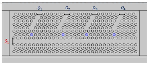
شکل (۹): ساختار دی‌مالتی پلکسر ۱×۴ پیشنهادی با شبکه مثلثی. استوانه‌های رنگی در مسیرهای خروجی یک تا چهار با ماده ENE پر شده و شعاع آنها به ترتیب عبارتند از: ۰/۹۶r، ۰/۹۷r، ۰/۹۸r و ۰/۹۹r.
