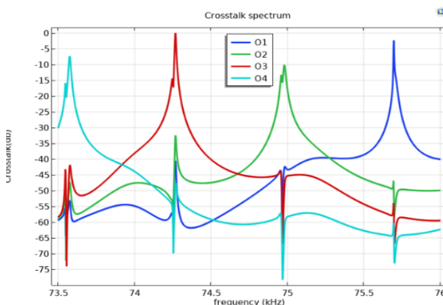
شکل (۱۱): منحنی‌های هم‌شنوایی دی‌مالتی‌پلکسر ۱×۴ پیشنهادی با شبکه‌ی مثلثی
