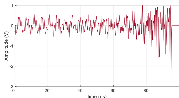
شکل (۵): سیگنال معکوس جهت بازتوزیع به محیط
