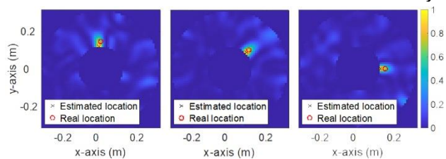
شکل (۱۴): برش عرضی توزیع شدت میدان الکتریکی در لحظات بازتمرکز امواج در سناریو ۴ (تخلیه جزئی چندگانه غیرهمزمان در سه مکان مختلف)
