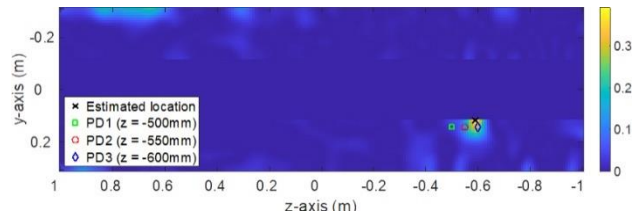
شکل (۱۵): تخلیه‌های جزئی چندگانه همزمان در سه مکان مختلف در طول محور Z (نتایج حاصل از معیار کمینه آنتروپی)
