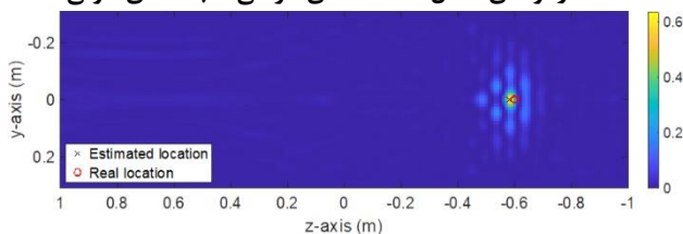
شکل (۷): برش طولی توزیع لحظه‌ای شدت میدان الکتریکی در لحظه بازتمرکز امواج (لحظه دارای کمینه آنتروپی) در سناریو ۱
