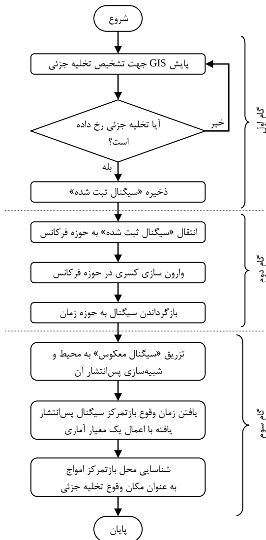
شکل (۲): فلوچارت مکان یابی تخلیه جزئی به روش فیلتر معکوس
