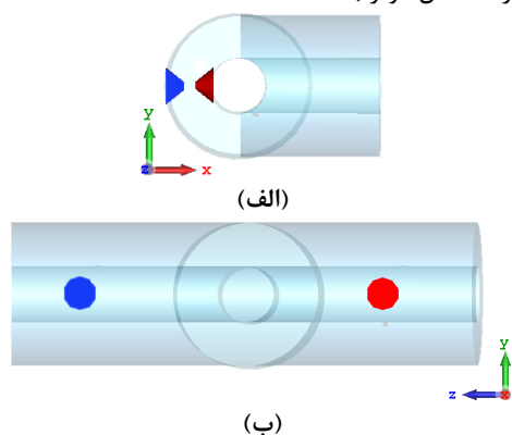
شکل (۹): جانمایی سنسور (آبی رنگ) و تخلیه جزئی (قرمز رنگ) در ساختار T شکل؛ (الف): نمای عرضی؛ (ب): نمای طولی
