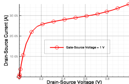
شکل (۱۸): نمودار جریان درین_سورس برحسب ولتاژ درین_سورس
