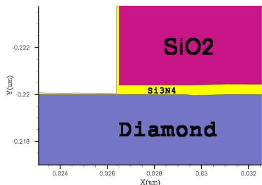
شکل (۸): لایه‌نشانی Si 3 N 4 بر روی عایق های ترانزیستور
