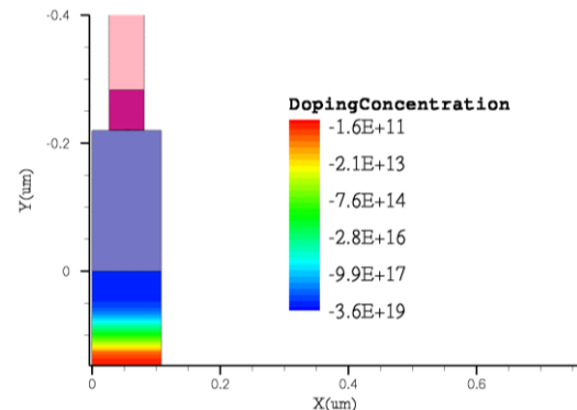
شکل (۶): زدایش نواحی اضافی عایق دوم (اکسید سیلیکون)
