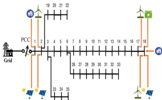
شکل (۷): تعداد و محل بهینه نصب DERها با افزایش در نرخ وقوع سوانح
