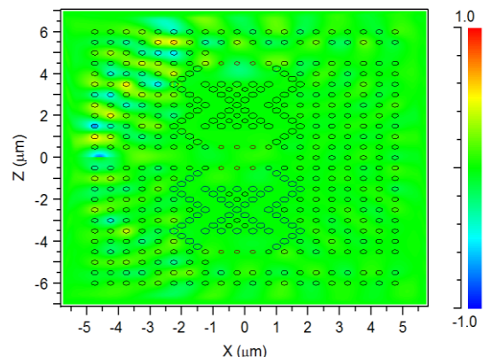
شکل (۳): نحوه توزیع میدان در \lambda=1000nm
