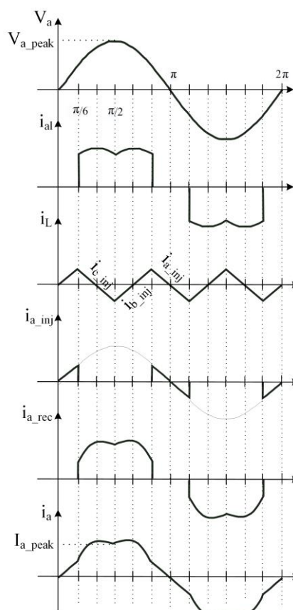
شکل (۴): شکل موج های یکسوساز فعال تزریق هارمونیک سوم GPU
