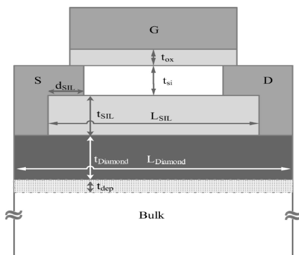
شکل (۱): ساختار ماسفت سیلیکون روی الماس با عایق دولایه بدنه فوق نازک [۱۴]
