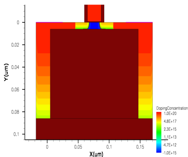
شکل (۳): افزاره‌ی سیلیکون بر روی الماس دو لایه عایق در حالت کمینه
