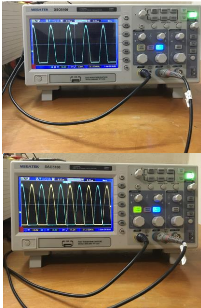
شکل (۱۰): شکل بالا نمونه سیگنال ولتاژ پایه درین ماسفت M_1 ، شکل وسط نمونه سیگنال ولتاژ پایه درین ماسفت M_2 ، و شکل پایین ولتاژ پایه‌های درین ماسفت‌های M_1 و M_2 با هم در اسیلوسکوپ
