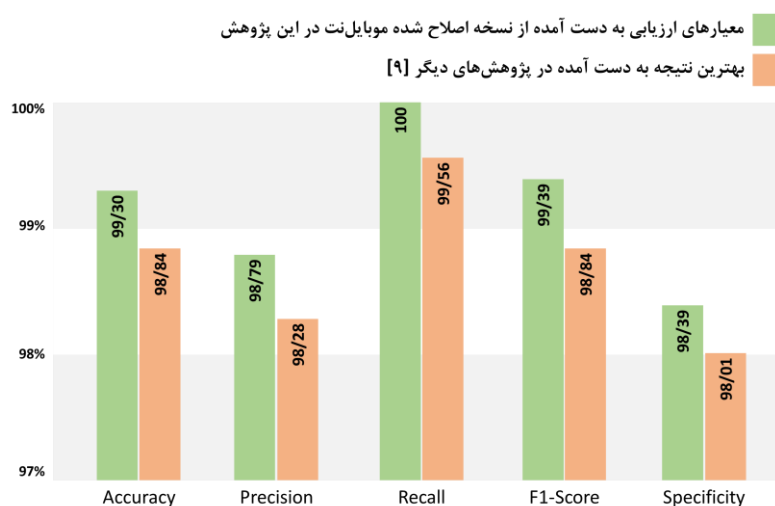
شکل (۱۰): مقایسه نتیجه معیارهای ارزیابی حاصل از روش پیشنهادی با بهترین مدل پژوهش‌های دیگر
