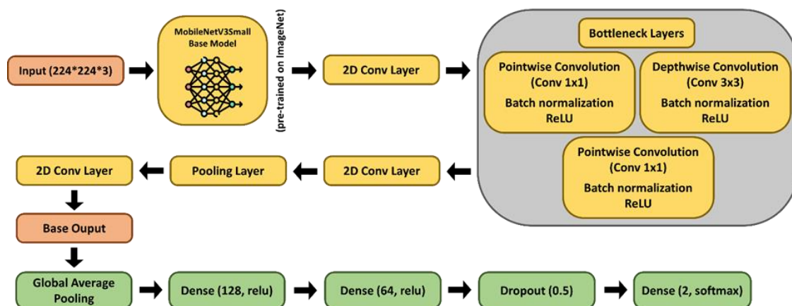
شکل (۵): فلوچارت معماری نسخه بهبود یافته موبایل‌نت
