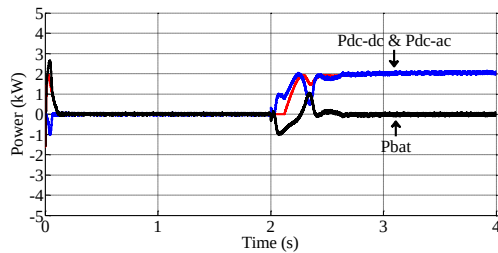
شکل (۱۶): توان مبدل dc-dc، dc-ac و شارژ باتری در آزمایش ۲
