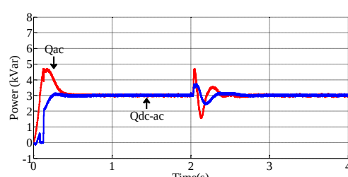
شکل (۲۰): توان راکتیو مبدل dc-ac و ریزشبه‌ی AC در آزمایش ۳
