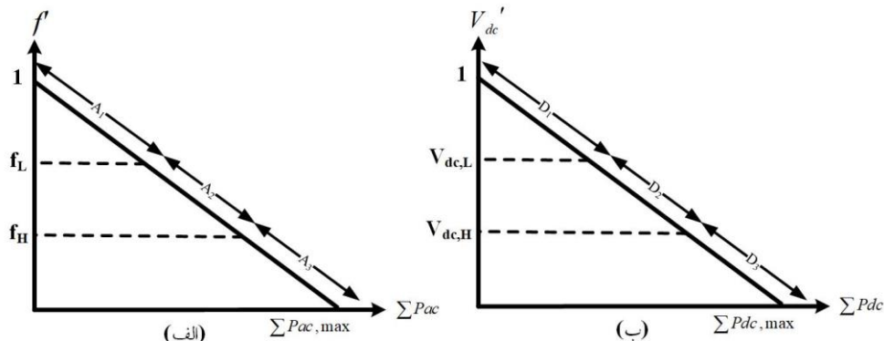
شکل (۶): منحنی افقی تجمعی منابع ریزشبهی AC و ریزشبهی DC
