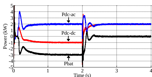
شکل (۲۲): توان مبدل dc-dc، dc-ac و شارژ باتری در آزمایش ۴
