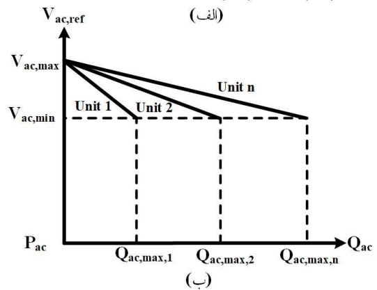
شکل (۴): منحنی افتی منابع ریزشبهی AC
