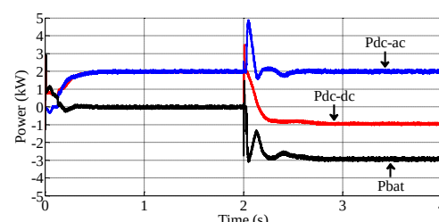
شکل (۱۹): توان مبدل dc-dc، dc-ac و شارژ باتری در آزمایش ۳
