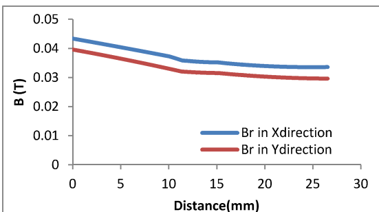
شکل (۱۳): مولفه‌ی چگالی شار عرضی در راستای X, Y در سیم پیچ HV ترانسفورماتور آوال
