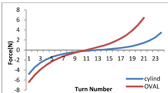
شکل (۱۲): نیروی محوری سیم پیچ LV در حالت عملکرد نرمال ترانسفورماتورهای آوال و سیلندری
