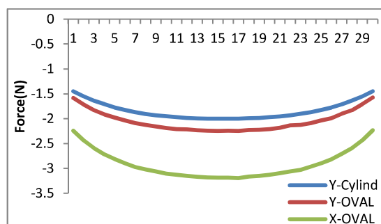
شکل (۱۰): مولفه‌ی X, Y نیروی شعاعی سیم پیچ HV در حالت عملکرد نرمال ترانسفورماتورهای آوال و سیلندری
