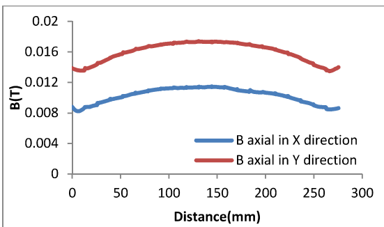
شکل (۱۱): مولفه‌ی چگالی شار محوری در راستای X, Y در سیم پیچ LV ترانسفورماتور آوال
