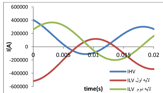
شکل (۱۴): منحنی جریان سیم پیچ‌های ترانسفورماتور اوال و سیلندری در شرایط اتصال کوتاه
