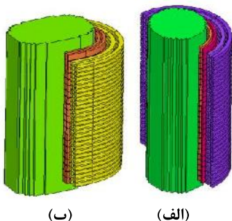
شکل (۵) مدل یک ساق ترانسفورماتور (الف) سیلندری (ب) اوال
