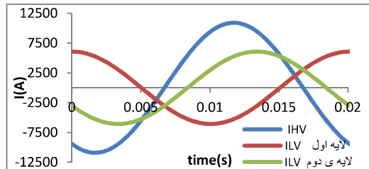
شکل (۴): منحنی جریان سیم پیچ های ترانسفورماتور اوال و سیلندری در شرایط عملکرد نرمال
