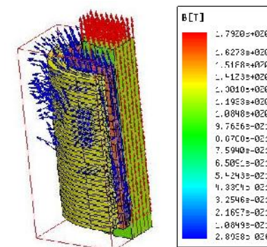
شکل (۷): بردارهای چگالی شار مغناطیسی ترانسفورماتور اوال
