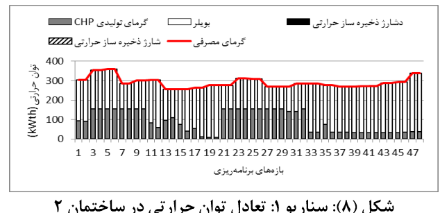
شکل (۸): سناریو ۱: تعادل توان حرارتی در ساختمان ۲
