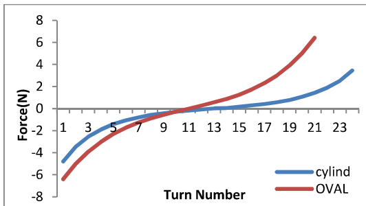
شکل (۱۲): نیروی محوری سیم پیچ LV در حالت عملکرد نرمال ترانسفورماتورهای اوال و سیلندری
