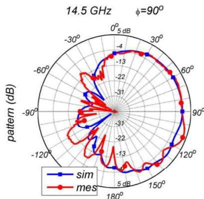
شکل (۲۰): الگوی تشعشعی آنتن در صفحه‌ی \phi=90^\circ در 14.5 GHz
