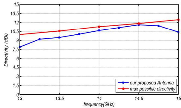
شکل (۱۷): نمودار مقایسه‌ی جهت‌دهی آنتن طراحی شده و حداکثر جهت‌دهی قابل دستیابی در جهت \theta=90^\circ و \phi=90^\circ جهت‌دهی آنتن در فرکانسی که لنز در آن طراحی شده است به حداکثر مقدار خود می‌رسد.
