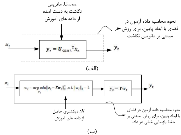
شکل (۲): بلوک دیاگرام محاسبه مختصات داده آزمون در فضای ابعاد پایین با روش پیشنهادی SRML، مبتنی بر ماتریس نگاشت (ب) مبتنی بر حفظ بازنمایی خطی هر داده.
