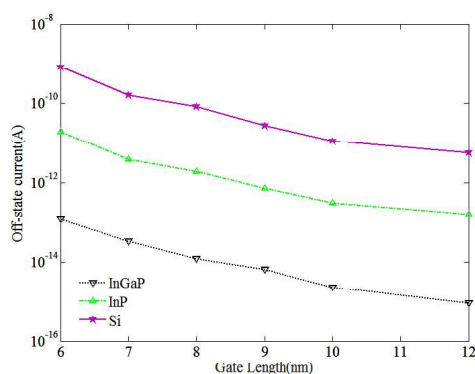
شکل (۵): نمودار جریان حالت خاموش ترانزیستورهای بدون پیوند با مواد کانال InGaP, InP و Si در طول گیت‌های ۶ تا ۱۲ نانومتر.
