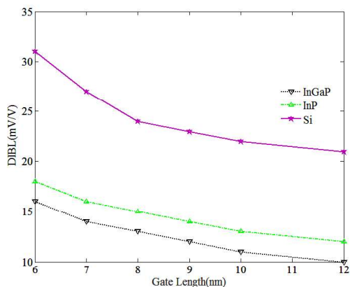
شکل (۸): نمودار دیبل ترانزیستورهای بدون پیوند با مواد InGaP, InP و Si در طول گیت‌های ۶ تا ۱۲ نانومتر.
