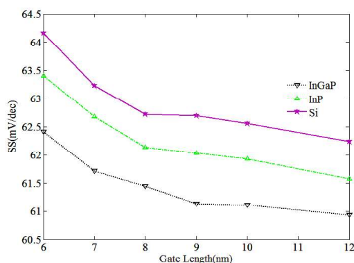
شکل (۷): نمودار شیب زیر آستانه ترانزیستورهای بدون پیوند با مواد InGaP, InP و Si در طول گیت‌های ۶ تا ۱۲ نانومتر.
