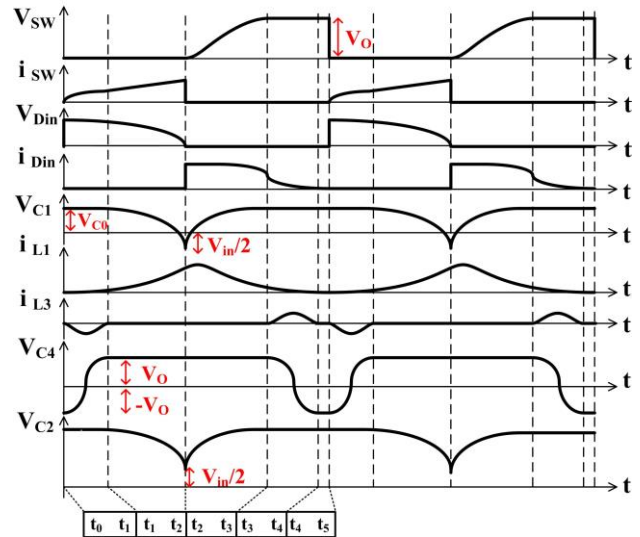
شکل (۲): شکل موج های تئوری مبدل شبه منبع امپدانس پیشنهادی
