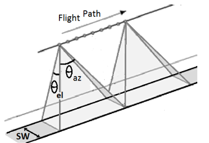
شکل (۱): هندسه مسیر تصویربرداری و زوایای پرتو نیم توان آنتن
