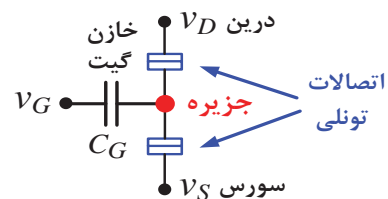
شکل (۱): آرایش مداری یک ترانزیستور SET
