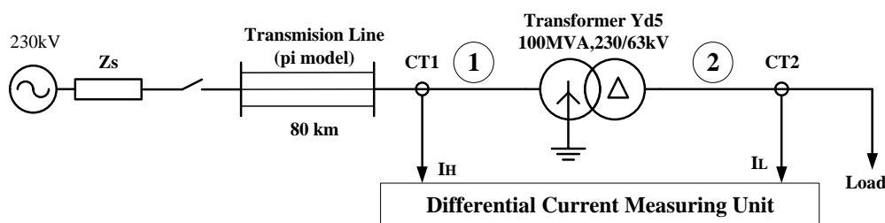
شکل (۲): دیاگرام سیستم قدرت شبیه‌سازی شده
