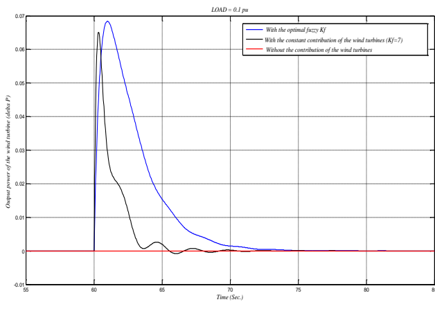
شکل (۱۵): دینامیک توان خروجی توربین‌های بادی سرعت متغیر الف) با حلقه کنترل اینرسی فازی ب) با حلقه کنترل اینرسی ج) بدون حلقه کنترل اینرسی
