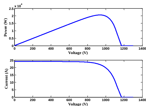
شکل (۷): نمودار مشخصه P-V و I-V برای ماژول PV
