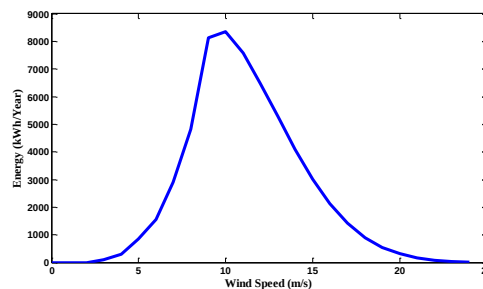
شکل (۵): انرژی خروجی کل توربین بادی برای یک سال
