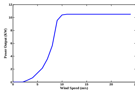
شکل (۴): منحنی توان توربین بادی ARE442
