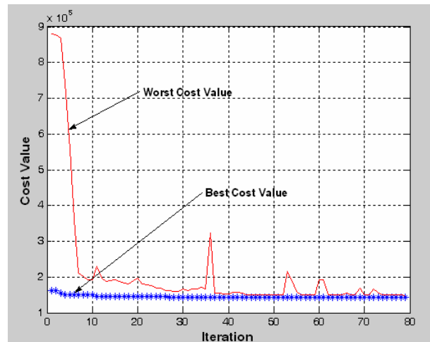
شکل (۱۰): هزینه بهینه شده بر حسب تعداد تکرار با نرخ واحد سوخت 0.5 [$/Lit]
