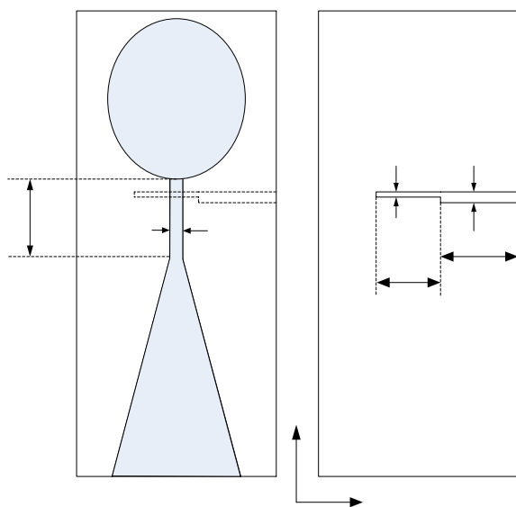
شکل (۵): ساختار آنتن TSA شبیه سازی شده
