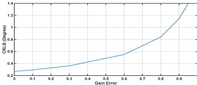
شکل (۹): مقدار CRLB(\theta) بر حسب مقادیر مختلف خطای بهره
