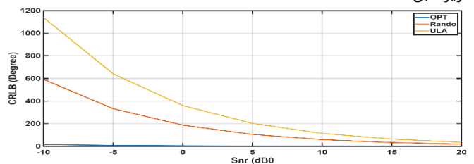
شکل (۷): مقدار CRLB(\theta) با وجود دو هدف بر حسب نسبت سیگنال به نویز
