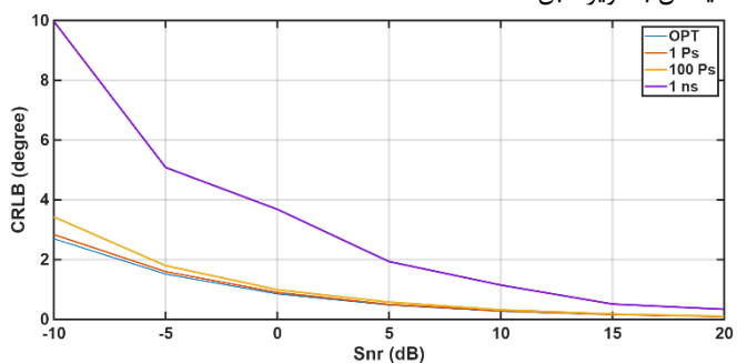
شکل (۱۱): مقدار \text{CRLB}(\theta) بر حسب مقادیر مختلف خطای
