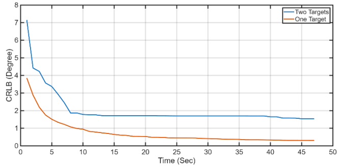
شکل (۵): مقدار CRLB(\theta) بر حسب گذر زمان در طول مسیر حرکت
