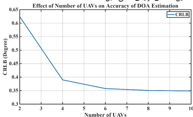
شکل (۲): مقدار CRLB(\theta) بر حسب تعداد پهپادها.
