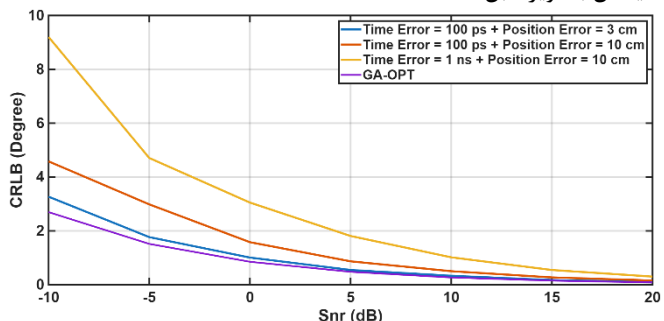
شکل (۱۲): مقدار \text{CRLB}(\theta) بر حسب مقادیر مختلف خطای
