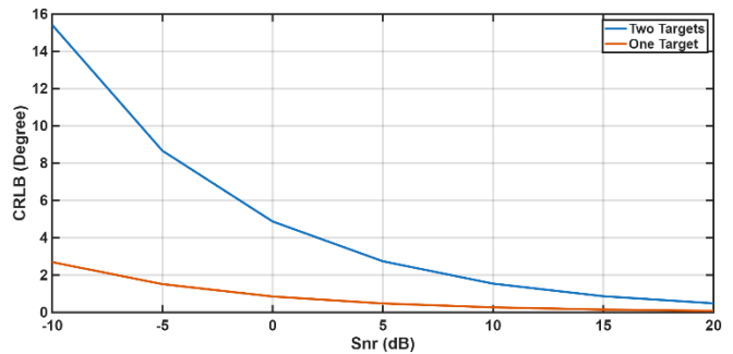
شکل (۶): مقدار CRLB(\theta) برای حالت بهینه با تعداد اهداف مختلف بر حسب نسبت سیگنال به نویز
