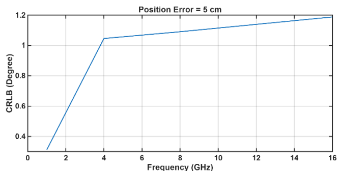
شکل (۱۴): مقدار CRLB(\theta) براساس رابطه‌ی (۴۰) با فرض وجود عدم قطعیت در موقعیت بر حسب فرکانس
