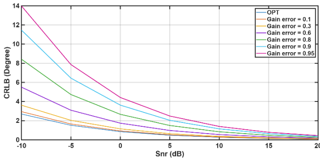
شکل (۸): مقدار CRLB(\theta) برای حالت بهینه و مقادیر مختلف خطای بهره بر حسب نسبت سیگنال
