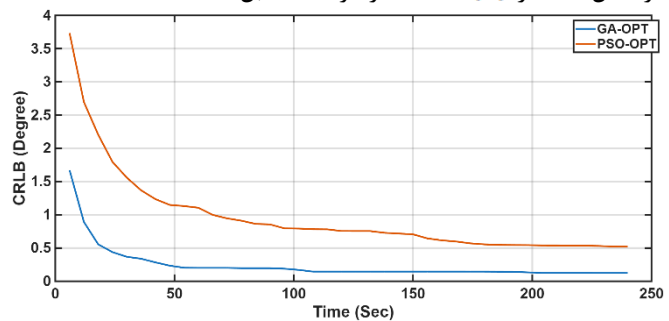
شکل (۳): مقدار CRLB(\theta) بر حسب گذر زمان در طول مسیر حرکت
