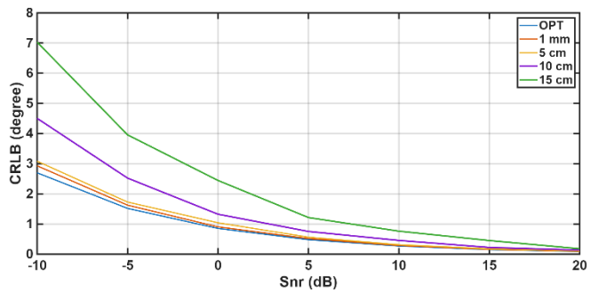
شکل (۱۰): مقدار \text{CRLB}(\theta) بر حسب مقادیر مختلف خطای موقعیت و حالت ایده‌آل بر حسب نسبت سیگنال به نویز
