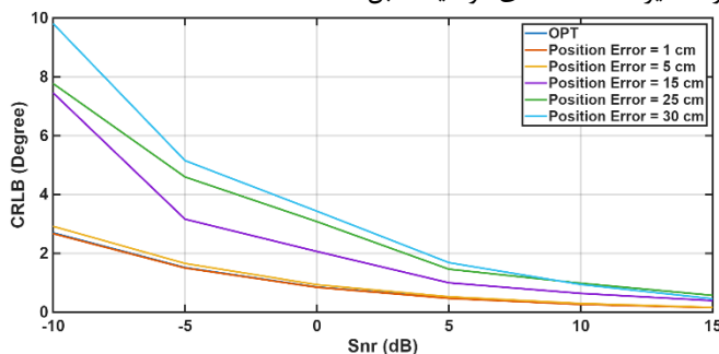
شکل (۱۶): مقدار CRLB(\theta) با در نظر گرفتن اثرات اغتشاشات پرواز
