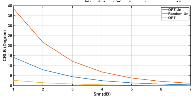
شکل (۱۳): مقدار \text{CRLB}(\theta) با فرض عوامل عدم قطعیت و مقدار \text{CRLB}(\theta) در حالت ایده‌آل بر حسب مقادیر مختلف نسبت سیگنال به نویز
