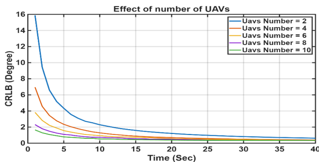
شکل (۱): مقدار CRLB(\theta) بر حسب گذر زمان در طول مسیر حرکت
