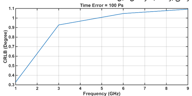
شکل (۱۵): مقدار CRLB(\theta) براساس رابطه‌ی (۴۰) با فرض وجود عدم قطعیت در همگام‌سازی زمانی بر حسب فرکانس
