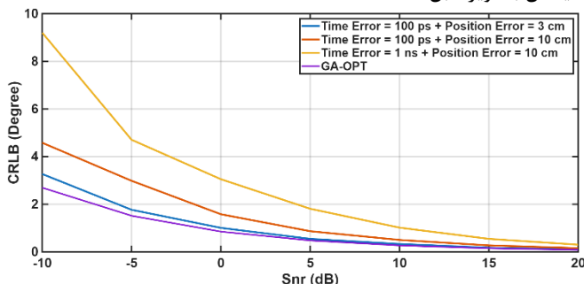
شکل (۱۲): مقدار \text{CRLB}(\theta) بر حسب مقادیر مختلف خطای
