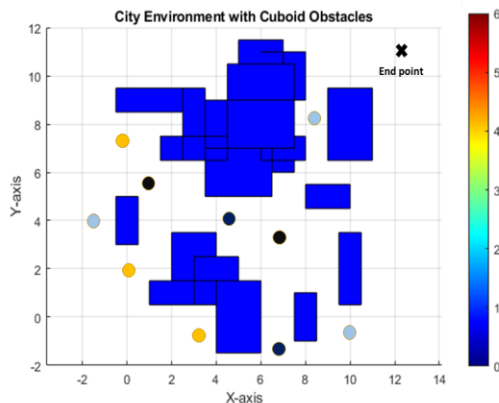
شکل (۴): اعمال خوشه‌بندی ایجاد شده پهبادهای ناهمگن به محیط غیر یکنواخت
