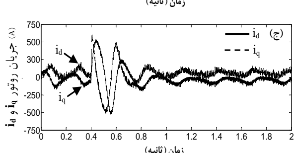
شکل (۷): نتایج شبیه‌سازی برای سرعت \pm 100 \text{ rpm} بدون جبران شار روتور، الف: پروفایل سرعت روتور، ب: پروفایل گشتاور تولیدی و ج: مؤلفه‌های جریان روتور در قاب dq
