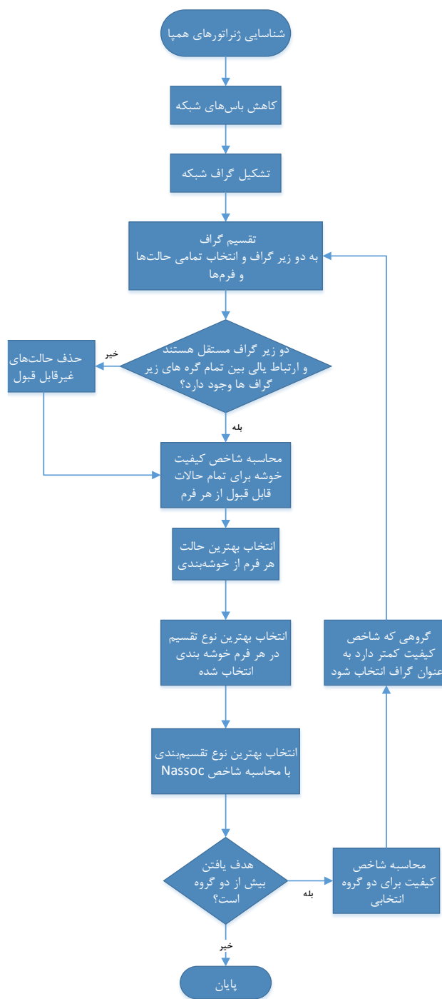
شکل (۴): فلوچارت الگوریتم پیشنهادی
