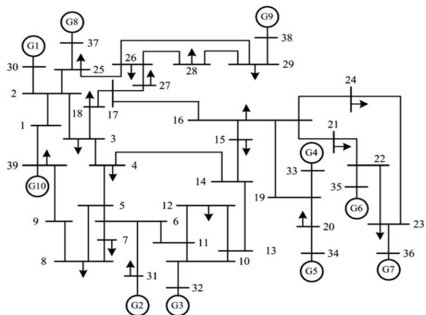
شکل (۵): شبکه ۳۹ باس IEEE
